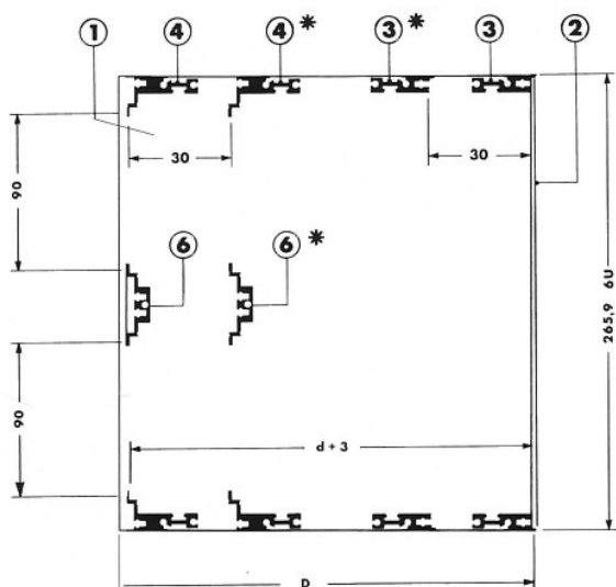
6U x 84HP Type 1 DIN 41612
